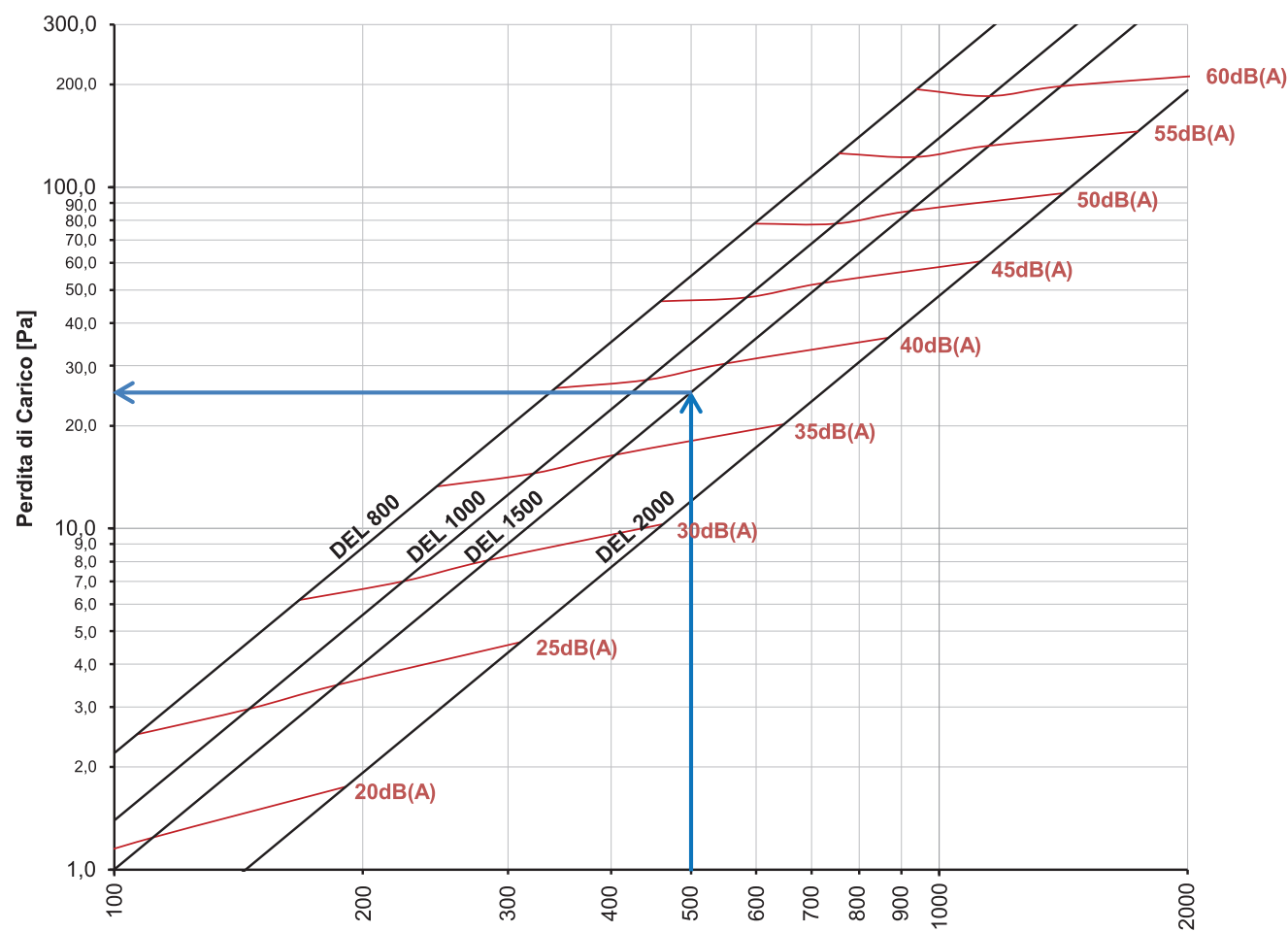
Portata / Perdita di Carico / Livello Acustico Modelli DEL - 3 SLOT
