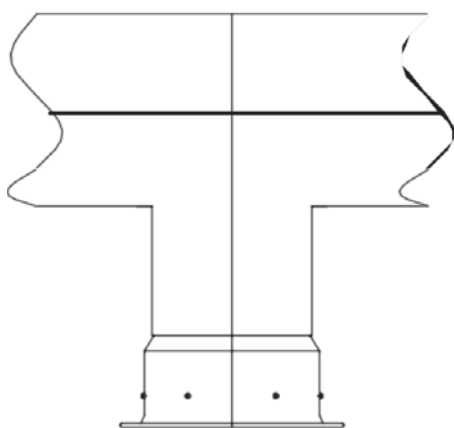
FIG.2 MONTAGGIO SU CANALE CON CANOTTO DI RACCORDO
