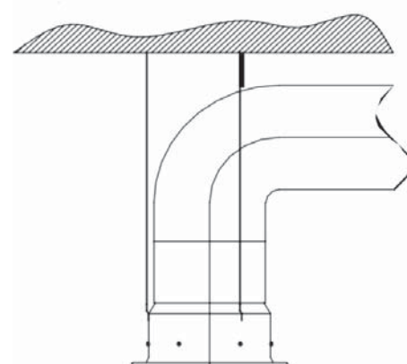
FIG.3 MONTAGGIO CON TUBO FLESSIBILE
