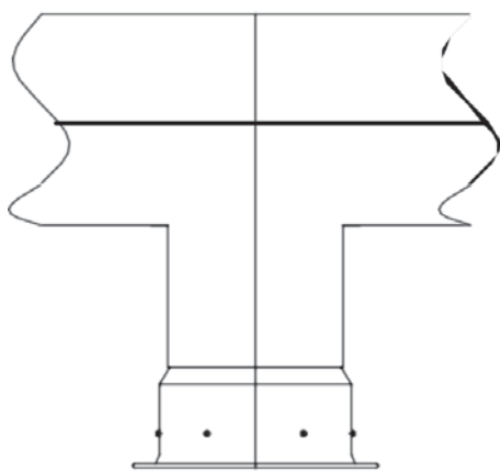
FIG.2 MONTAGGIO SU CANALE CON CANOTTO DI RACCORDO
